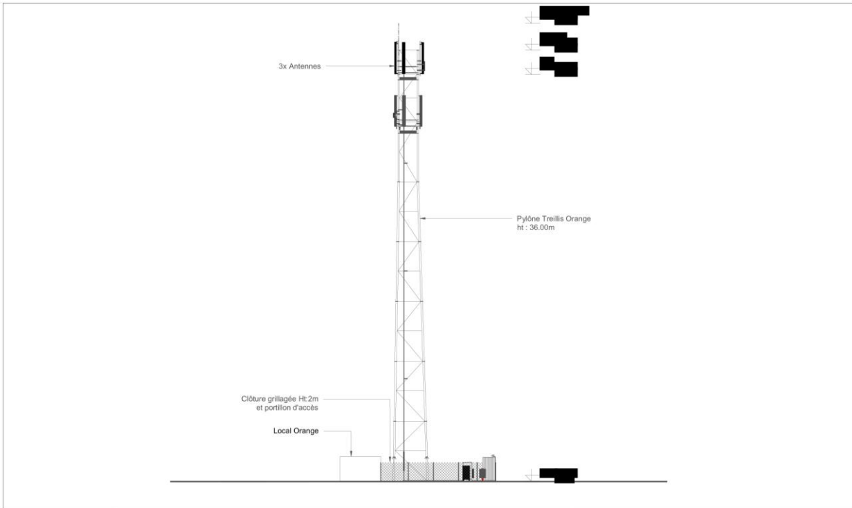
plan élévation
